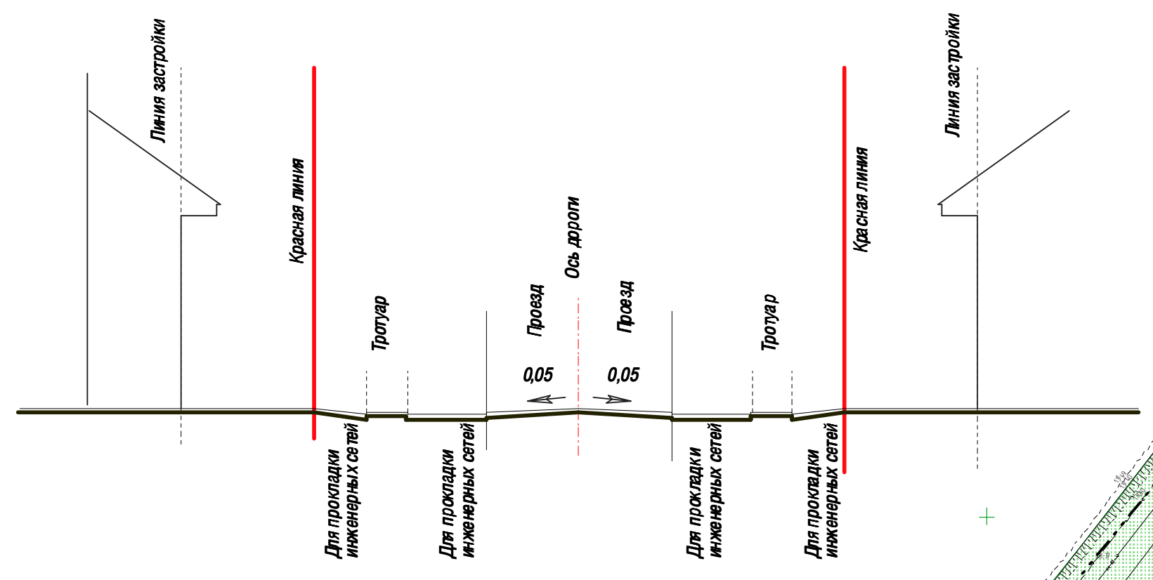
Поперечный профиль улиц, проездов
